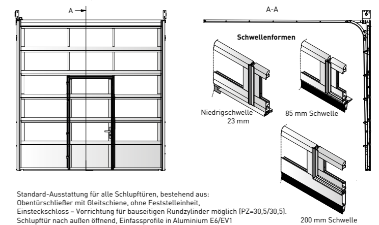
SL 40 mit Schluftpür (optional)
