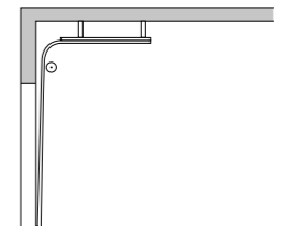
HLU: Höhergeführter Laufschienen-Beschlag mit untenliegender Torsionsfederwelle
