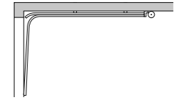
NSH: Niedrigsturz-Beschlag mit hintenliegender Federwelle
