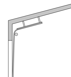
HLDU: Höhergeführter Laufschienen-Beschlag mit Dachfolge und untenliegender Torsionsfederwelle
