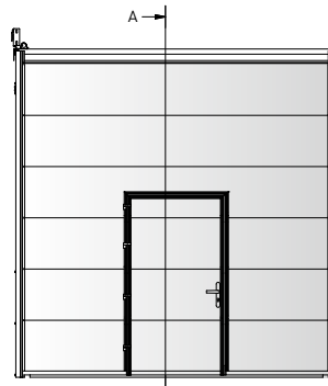
SW 40 mit Schlupftür (optional)
